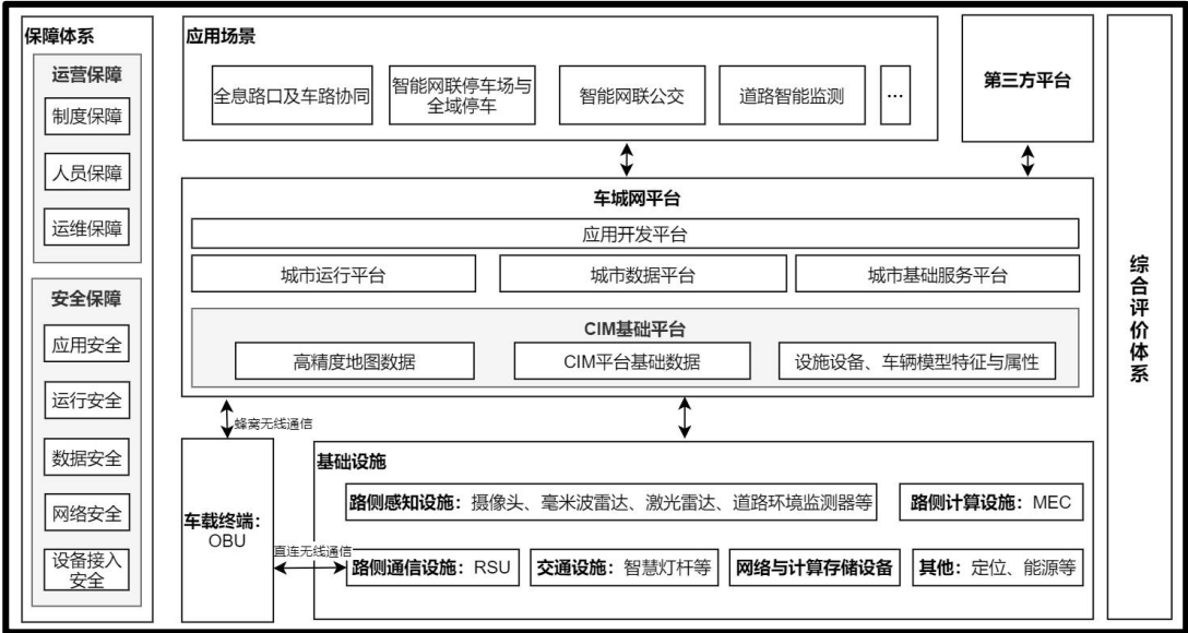
图1 车城网架构
